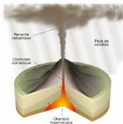
Eruption plinienne
