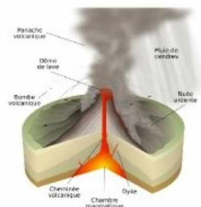
Eruption peléenne
