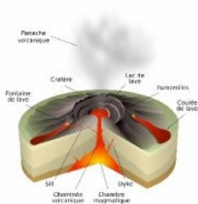
Eruption hawaïenne
